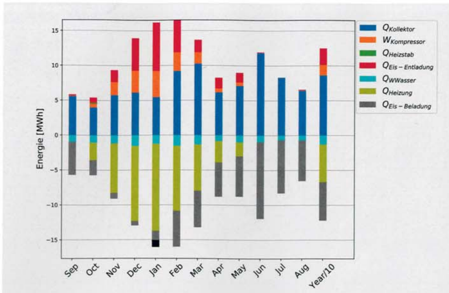
■ Monatliche Wärmebilanz der Solar-Eis-Heizung für das zweite Messjahr (September 2018 bis August 2019): Die roten Balken zeigen den Wärmeertrag aus dem Eisspeicher.
